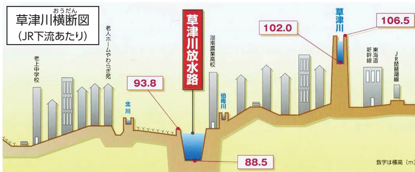
↑川の底が低くなった新しい草津川<草津川放水路工事記録誌より>
